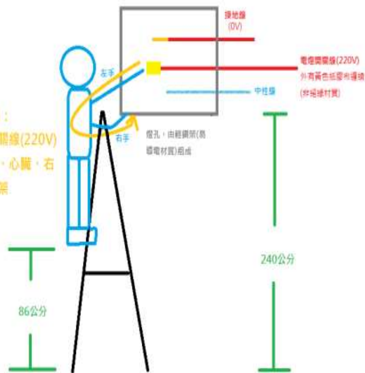
感電迴路示意圖
